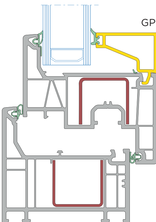
2fach Verglasung, eckige Glasleiste
