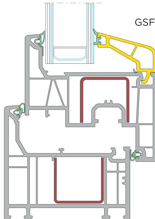
2fach Verglasung, abgerundete Glasleiste
