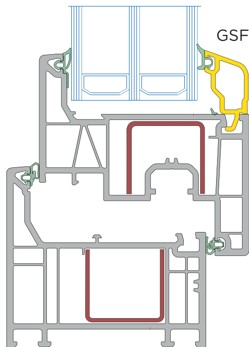
3fach Verglasung, abgerundete Glasleiste
