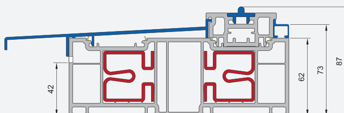
HSB 176 + HSB 276 mit Wetterschenkel
