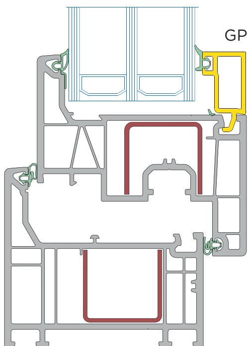
3fach Verglasung, eckige Glasleiste
