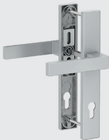
Drücker-Drücker Dublin37
